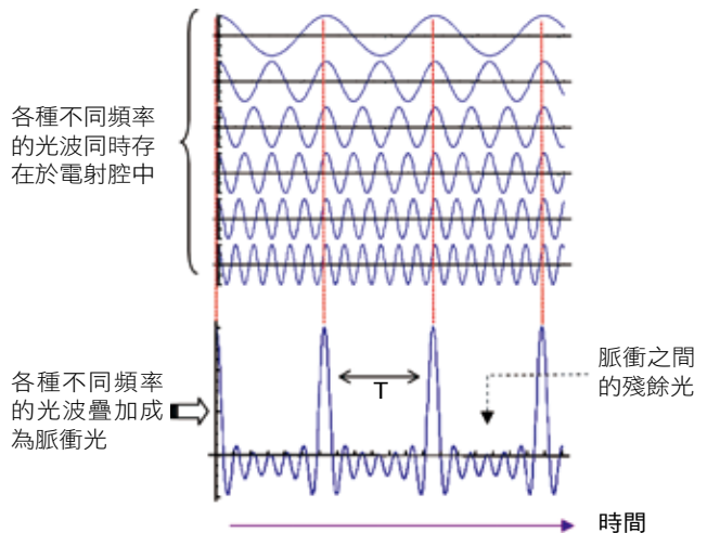
上面顯示6種雷射共振頻，當這6種光之間的相位是固定的，即波峰每隔一段時間會對齊一次，疊加起來便會形成下面的系列脈衝。
