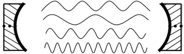
各種不同頻率的雷射光（符合共振腔駐波條件）同時輸出。
