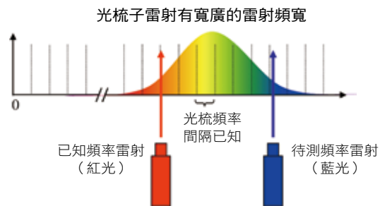
光梳子雷射的起初構想：用鎖模脈衝雷射與一個已知頻率雷射組成光梳雷射，鎖模脈衝雷射的間隔或光梳子雷射的頻率間隔，則由銫原子鐘決定。
